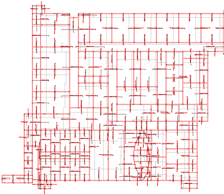
ARMADURA NEGATIVA DAS LAJES DO PAVIMENTO TERREO - NIVEL +0,00
