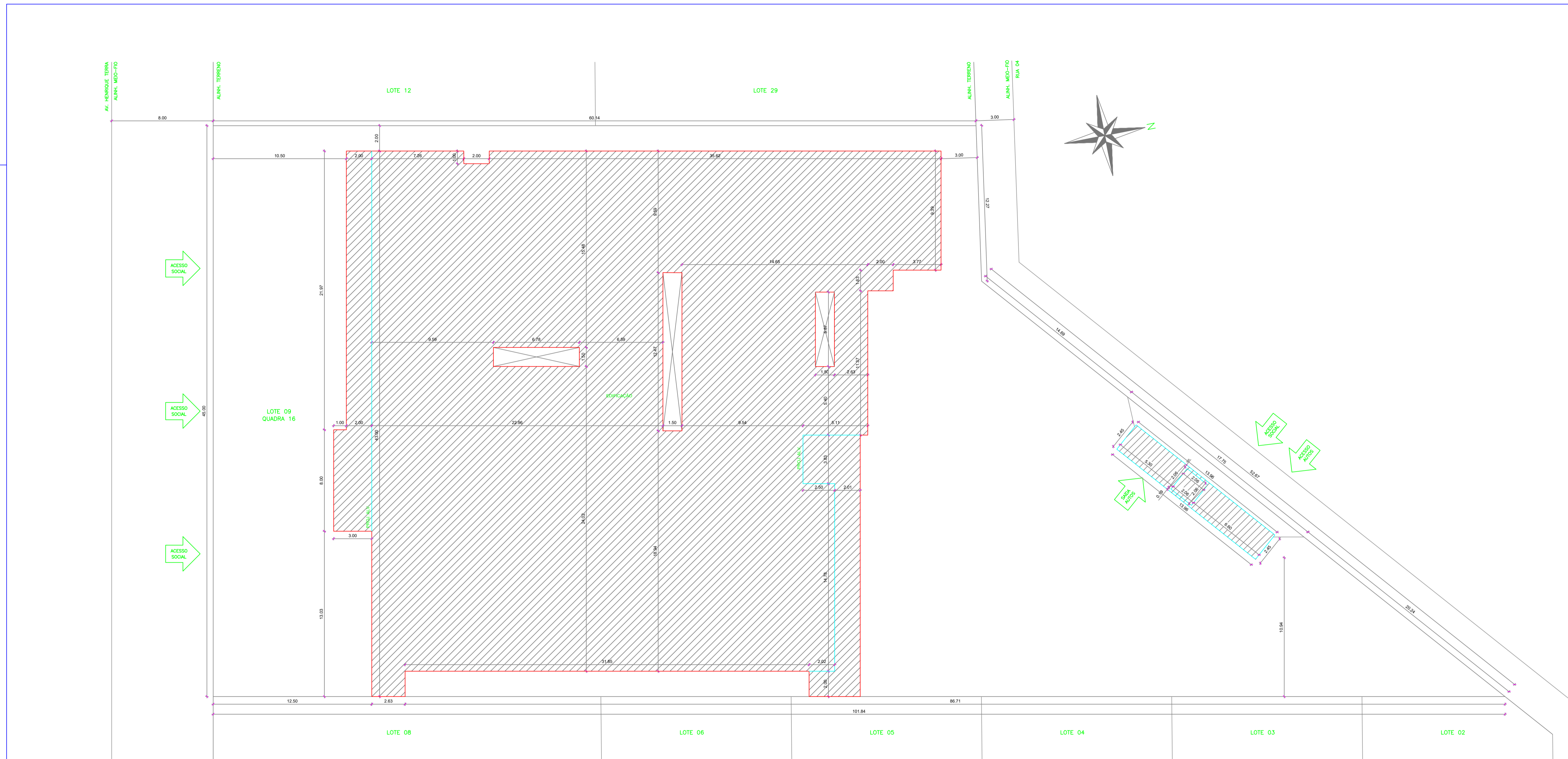
1 PLANTA DE SITUAÇÃO E IMPLANTAÇÃO esc.: 1/200
